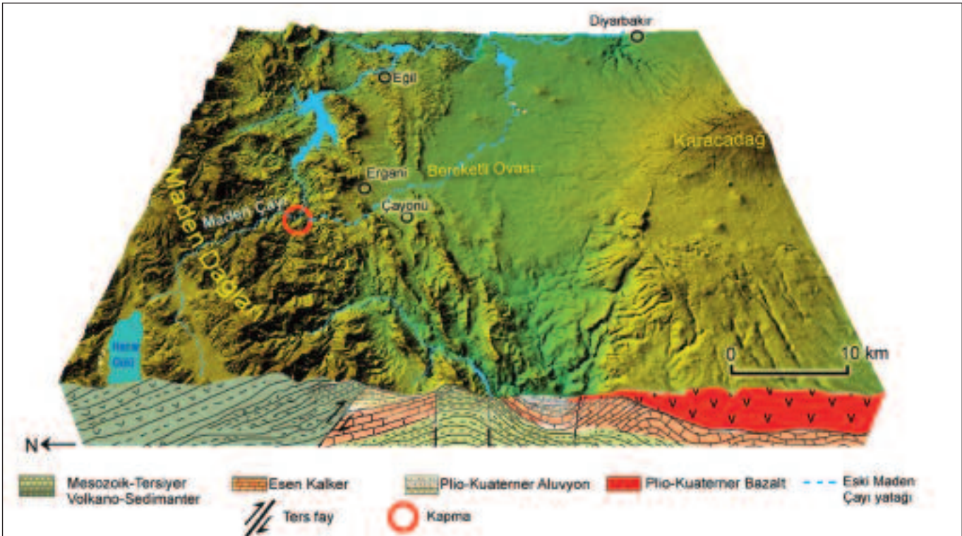
■ Şekil 5. Maden Çayı'nın orojenik yükselmeye yenik düşmesiyle yönünü doğuya çevirdiği, Fırat ve Dicle havzaları arasında yer alan ve Çayönü yerleşmesinin de kurulduğu su bölümü alanı üzerindeki yer süreçleri açısından sakin bir paleotopoğrafyayı gösteren blokdiyagram (Karadoğan ve Kuzucuoğlu, 2018).
