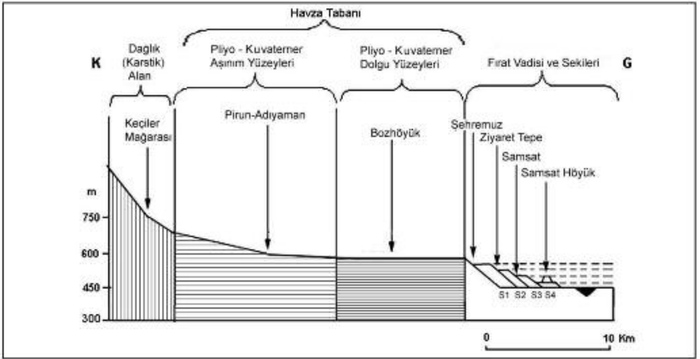
■ Şekil 2. Adıyaman havzasında Kuvaterner boyunca arazinin yarımla sürecine bağlı olarak yerleşmelerin gittikçe dikey yönde yer değiştirmesini gösteren kuzey-güney yönlü şematik kesit (Karadoğan ve Tonbul, 2007).
